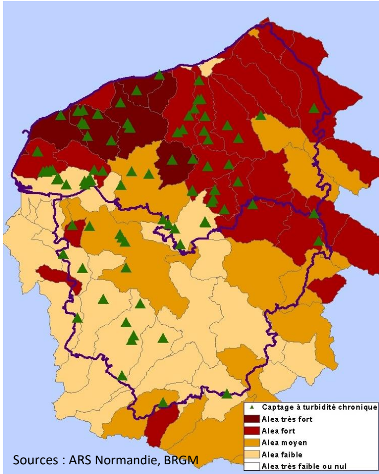
Aléa érosion et captages turbides (Haute-Normandie)
