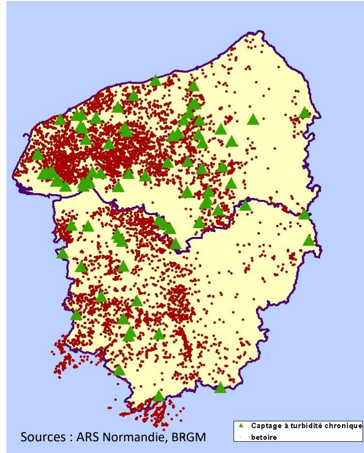
Karst et captages turbides (Haute-Normandie)
